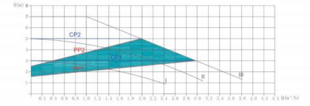
EBV-EC 25/7-130
