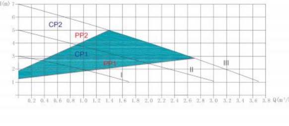
EBV32/7
