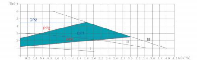
EBV-EC 32/6-180
