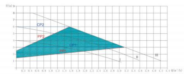
EBV-EC 25/8-180
