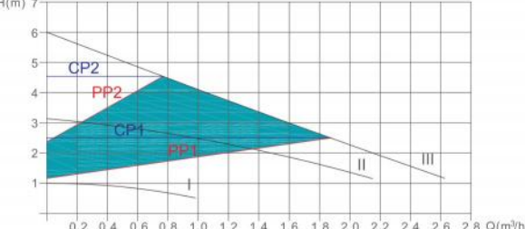
EBV15/6
