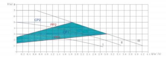
EBV-EC 32/7-180
