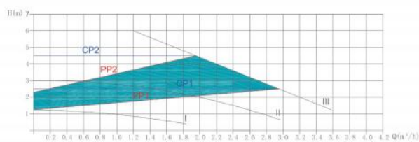
EBV-EC 25/6-130
