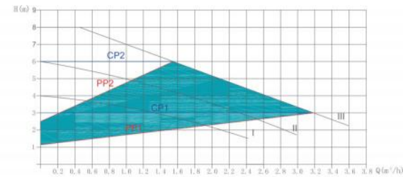
EBV-EC 25/8-180
