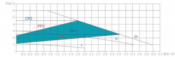
EBV-EC 25/6-180
