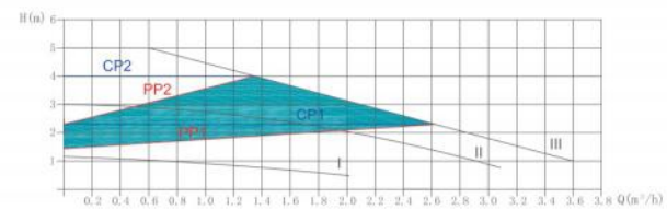
EBV-EC 32/5-180
