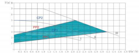
EBV-EC 15/7-130
