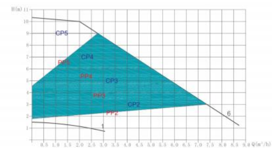
EBV-EB 32/10
