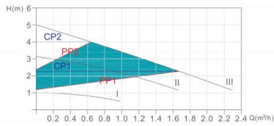
EBV15/5
