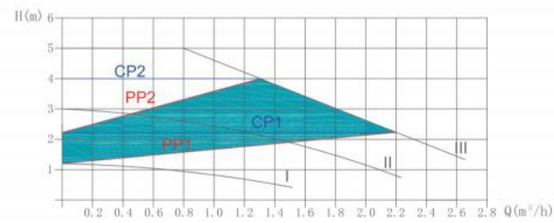
EBV-EC 15/5-130
