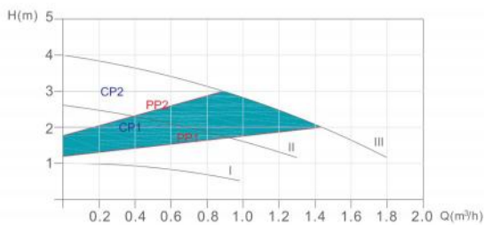
EBV15/4
