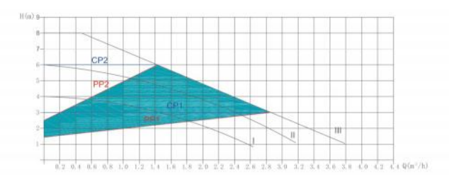
EBV-EC 25/8-130
