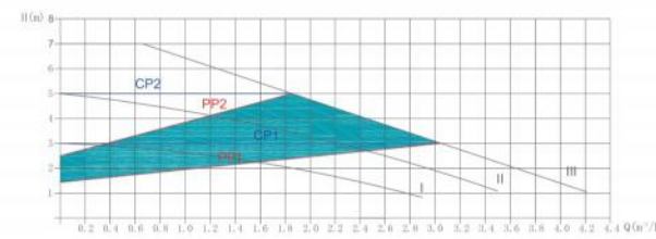
EBV-EC 25/7-180
